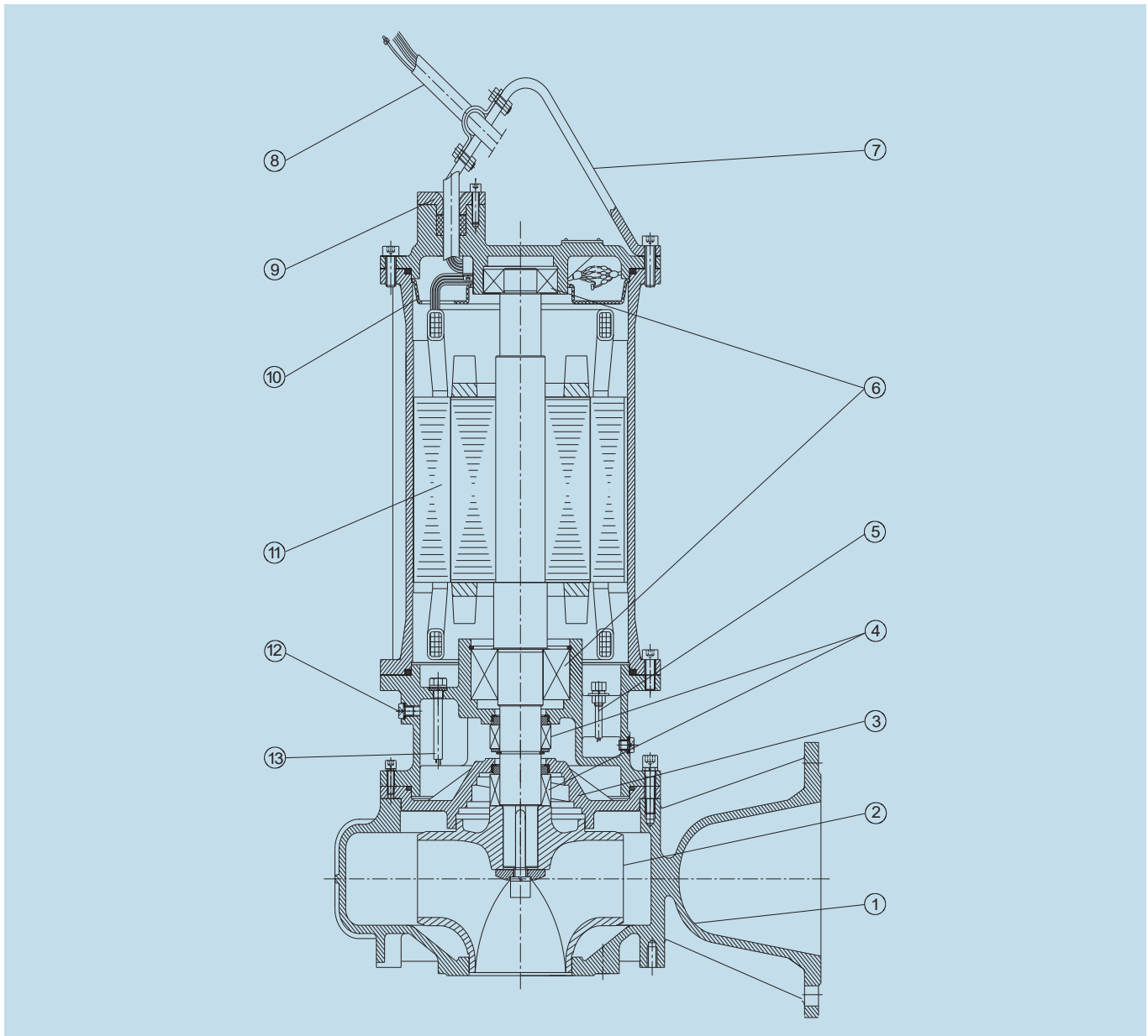
11kW-22kW Submersible Structural Diagram
