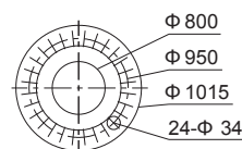
Discharge Flange
