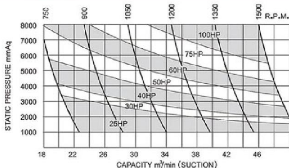
MODEL: DN-250(LT-250)
