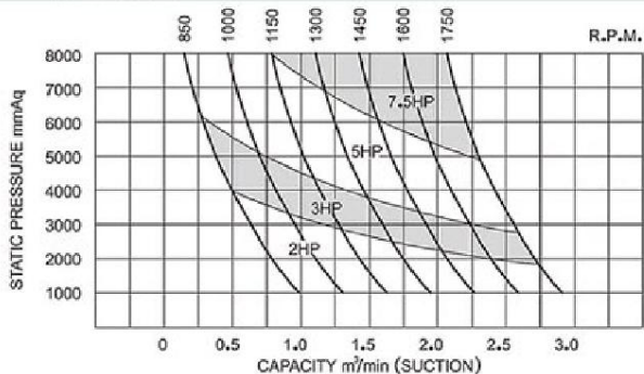
MODEL: DN-065(LT-065)
