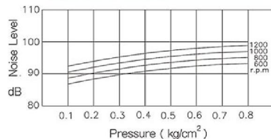
LT / LTV-300A
