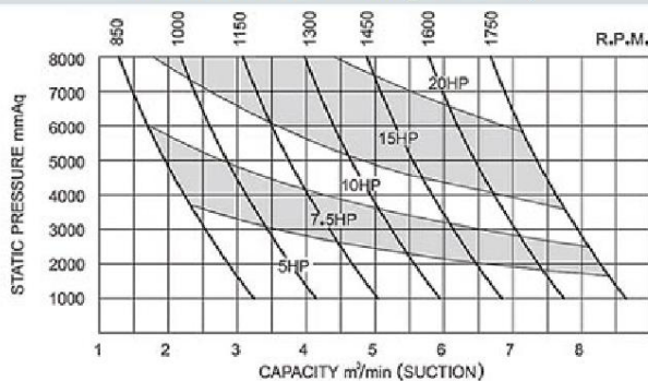
MODEL: DN-080(LT-080)
