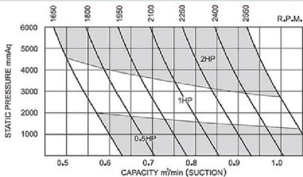
MODEL: DN-050(LT-050)
