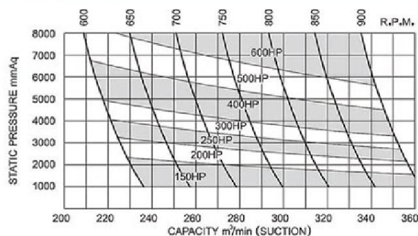
MODEL: DN-400(LT-400)
