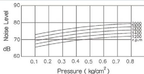
LT / LTV-050
