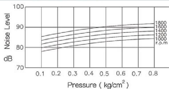
LT / LTV-125
