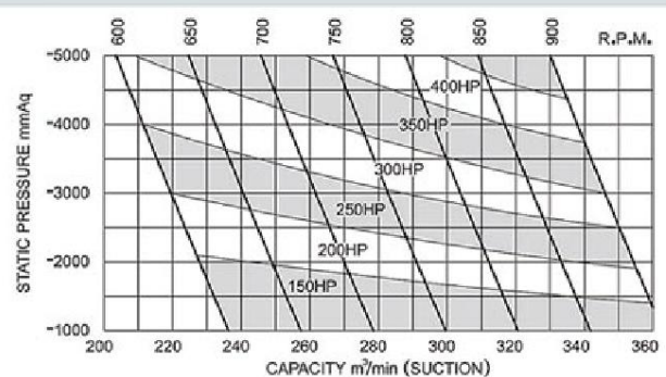
LTV-400
