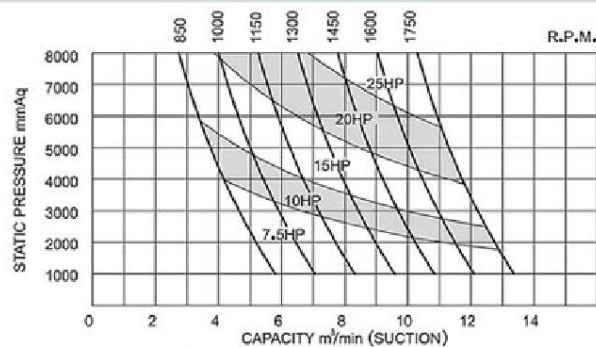
MODEL: DN-125S(LT-125S)
