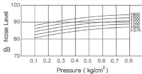
LT / LTV-150
