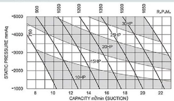
LTV-150
