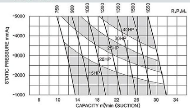
LTV-150
