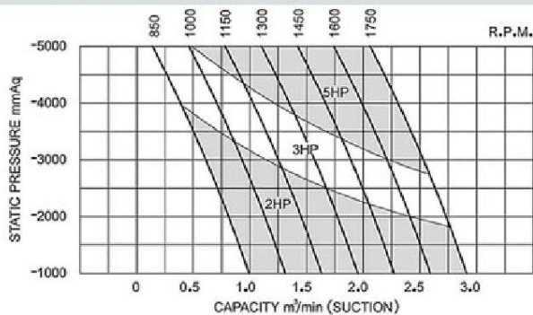
LTV-065
