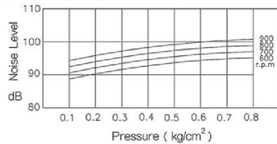
LT / LTV-400
