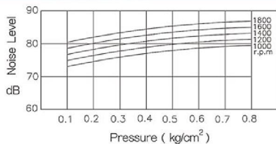
LT / LTV-080
