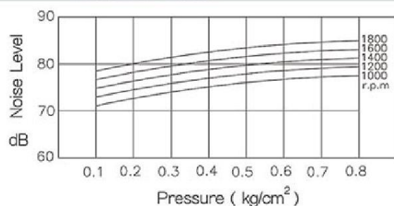
LT / LTV-065
