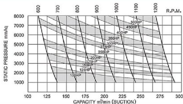
MODEL: DN-400(LT-400)
