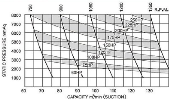
MODEL: DN-300(LT-300)
