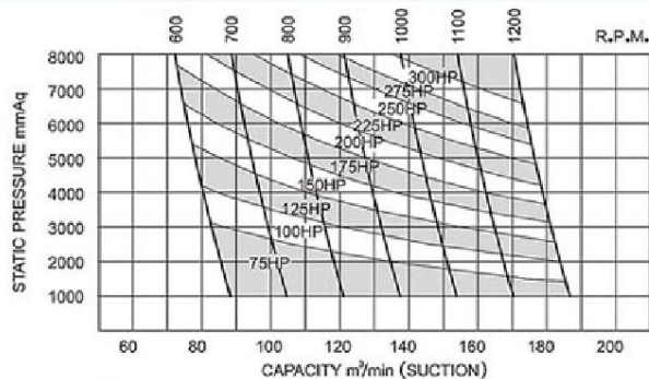
MODEL: DN-350(LT-350)
