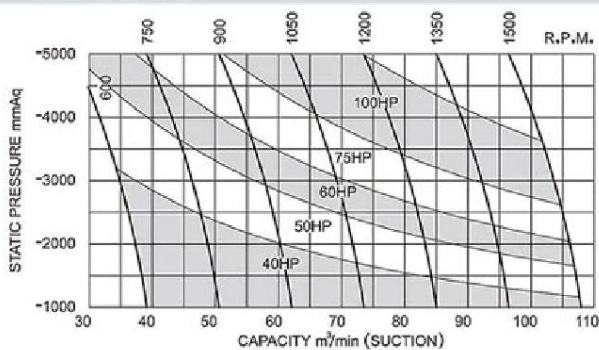
LTV-300
