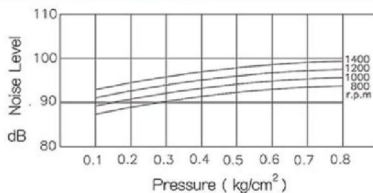
LT / LTV-300
