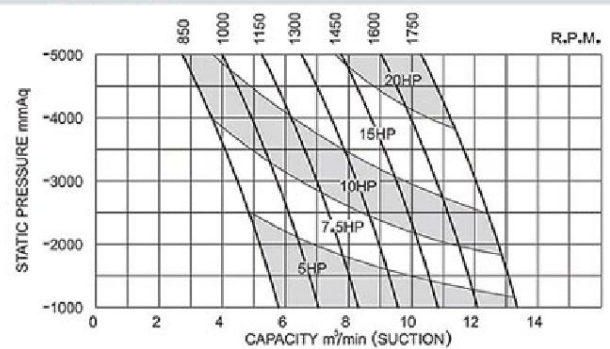
LTV-125S
