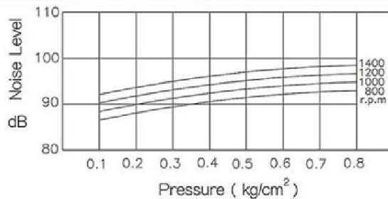
LT / LTV-250A
