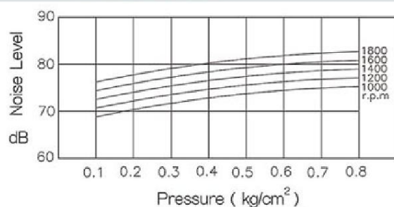
LT / LTV-065
