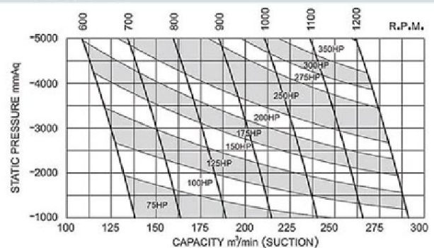
LTV-400
