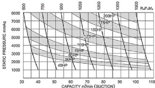
MODEL: DN-300(LT-300)
