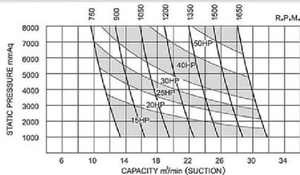
MODEL: DN-150(LT-080)
