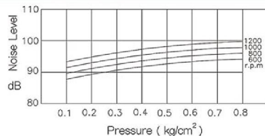
LT / LTV-350
