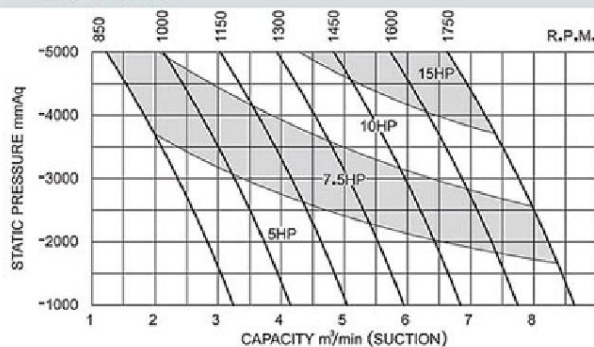
LTV-080
