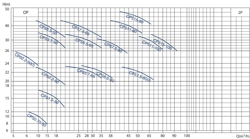
型谱图 Performance chart
