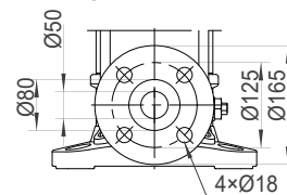
Flange PN25/DN25
